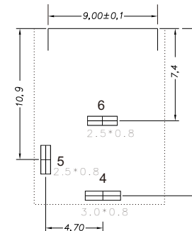
线路板开孔尺寸
